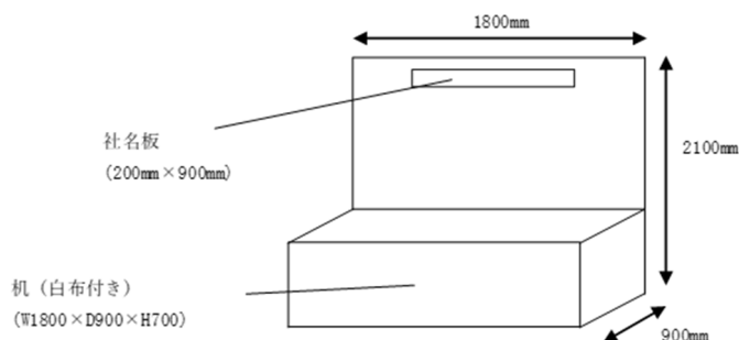
【基礎小間姿図：基礎小間仕様】
